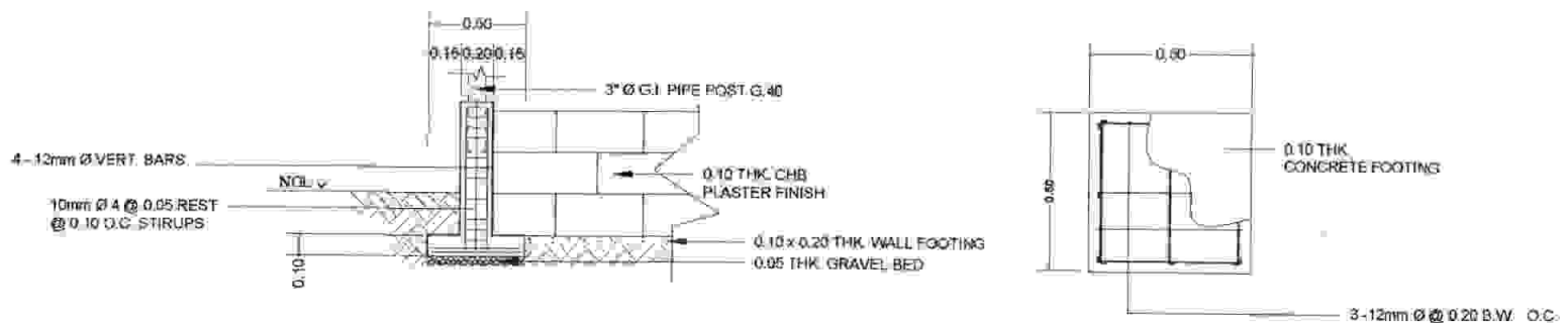
C1 / F1 DET.
