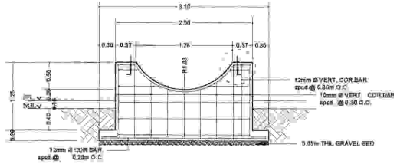
PEDESTAL DET.
